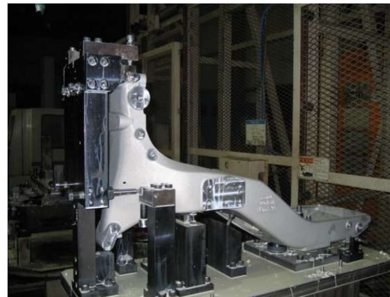
바이크 MAIN FRAME
